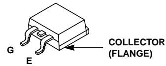
JEDEC TO-263AB
