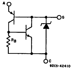
Fig. 23—Equivalent circuit.
