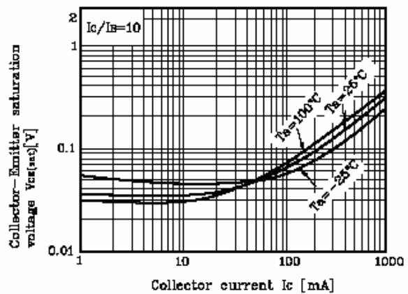
Fig. 4 V_{CE(sat)} - I_C
