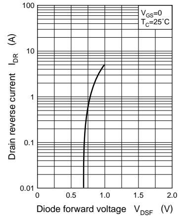
I_{DR} - V_{DSF}
