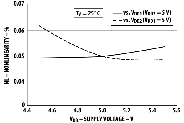
Figure 10 200-mV Nonlinearity vs. V DD1 and V DD2
