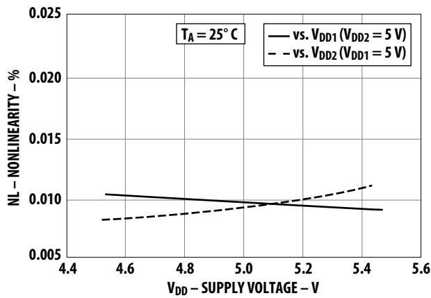
Figure 11 100-mV Nonlinearity vs. V DD1 and V DD2
