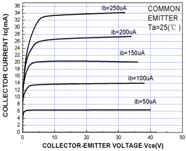
Ic-Vce
