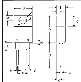
TO-220A
