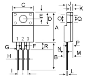
ITO-220AB
