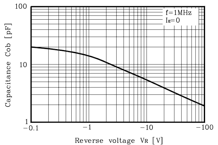
Fig. 4 C_{ob} - V_R
