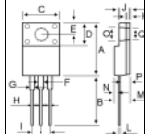
ITO-220
