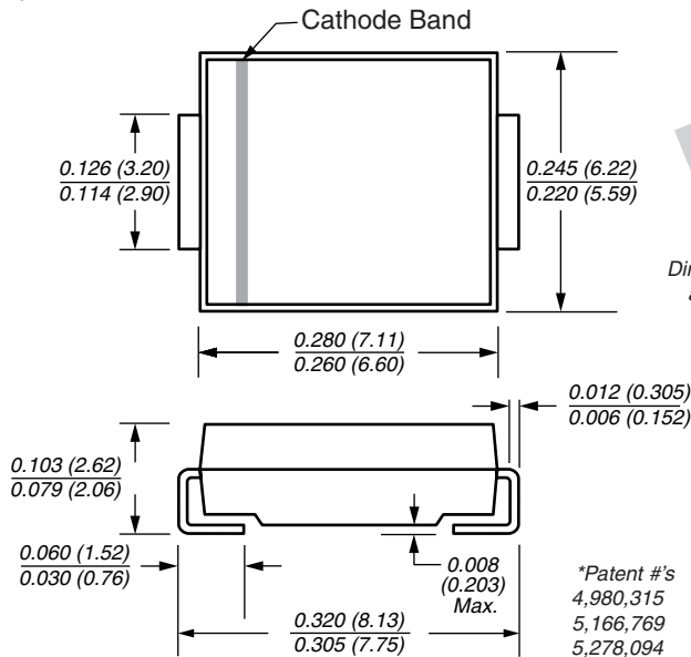
DO-214AB (SMC)
