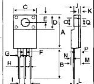
ITO-220
