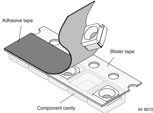
Fig. 12 - Blister Tape
