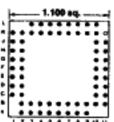
Footprint 11040
