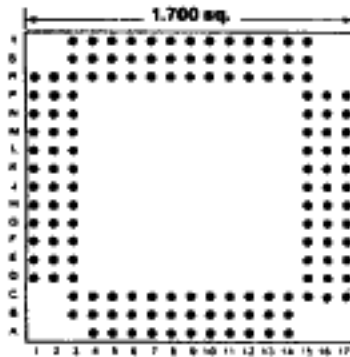
145 PINS Footprint 17004
