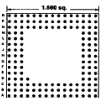
145 PINS Footprint 15024
