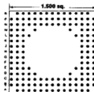
149 PINS Footprint 15019
