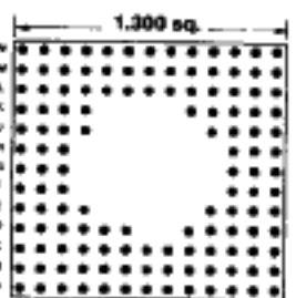
133 PINS Footprint 13048
