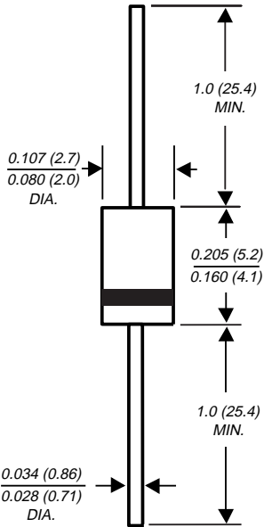
DO-204AL (DO-41)
