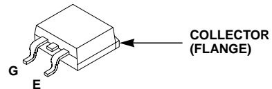
JEDEC TO-263AB
