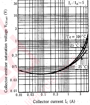
V_{CE(sat)} - I_C
