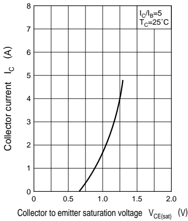
I_C - V_{CE(sat)}
