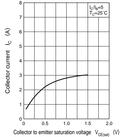
I_C - V_{CE(sat)}
