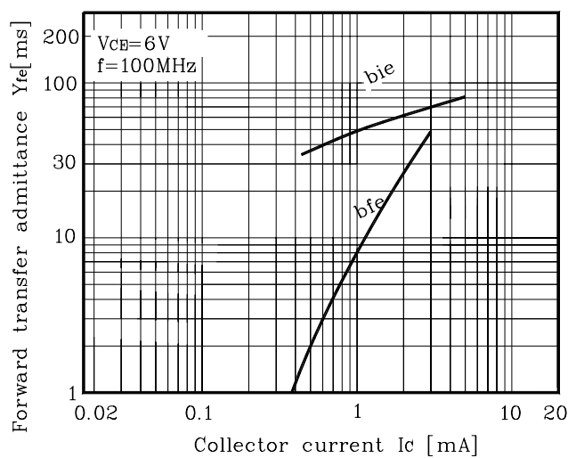
Fig. 8 I_C - Y_{fe}
