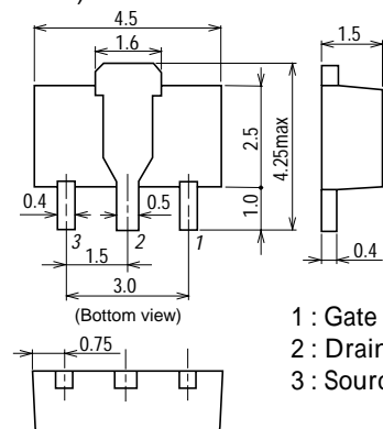
外形図 2062A
