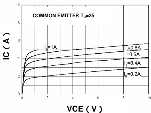
IC - VCE
