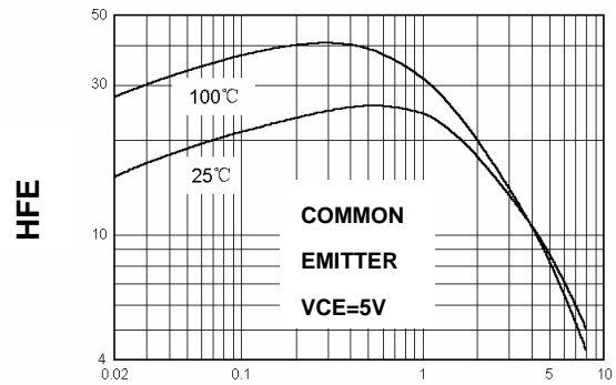
HFE - IC
