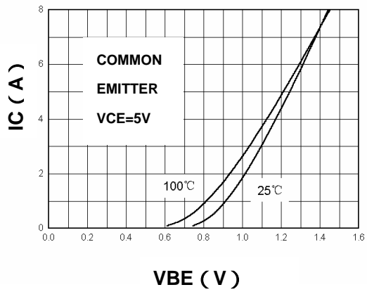
IC - VBE
