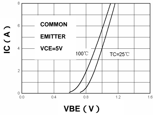
IC - VBE
