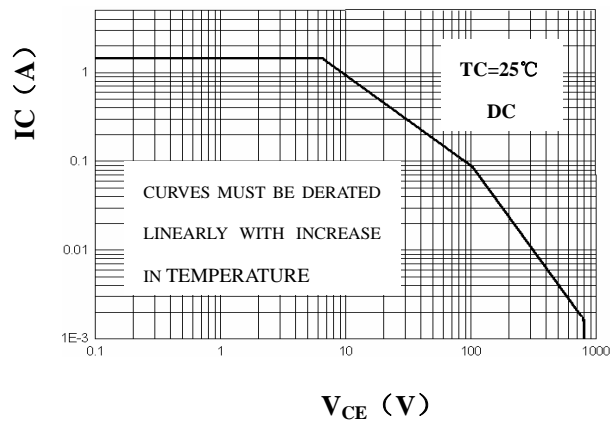
SOA
