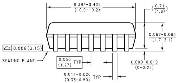
14-Lead Plastic EIAJ SOIC (SJ) Package Number M14D
