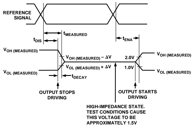
Figure 28. Output Enable/Disable
