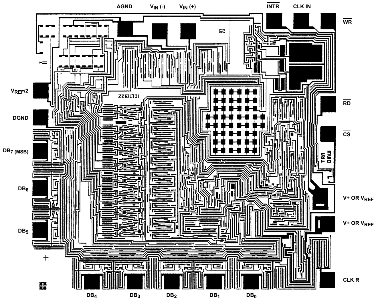
ADC0803, ADC0804
