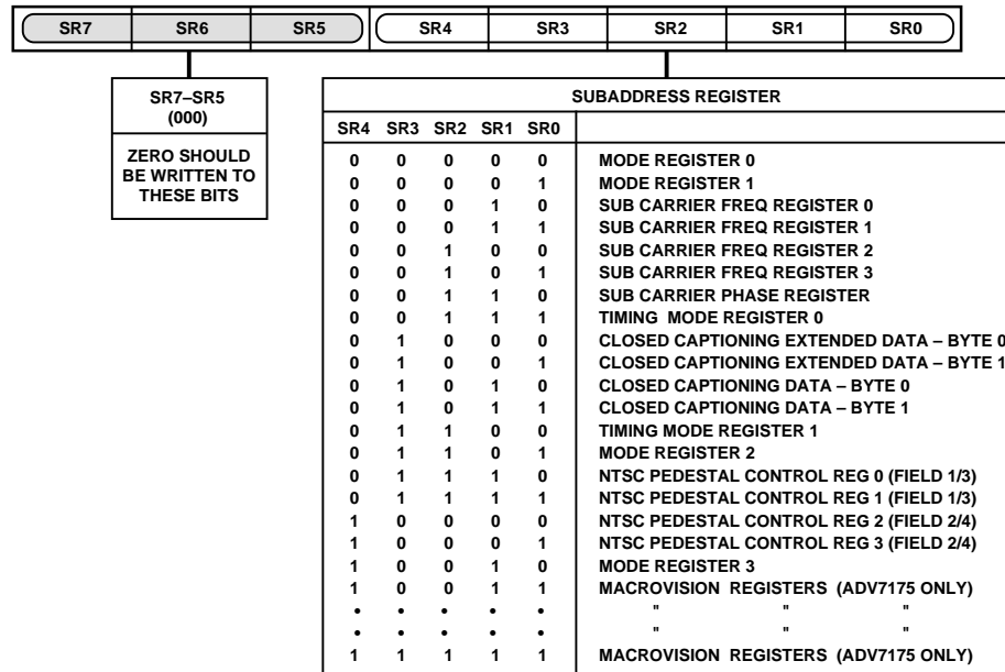
Figure 30. Subaddress Register
