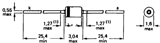
DO-34
