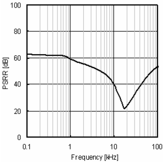
Fig.21 PSRR( I_o=0mA )
