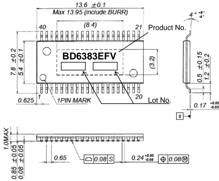
HTSSOP-B40 (Unit:mm)
