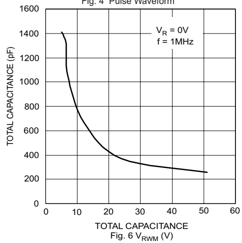
Fig. 6 V_{RWM} (V)
