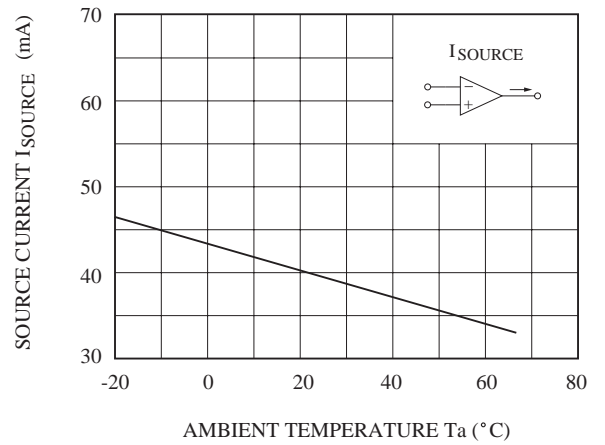
I_{SOURCE} - T_a
