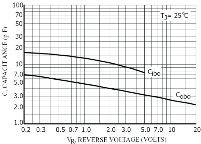
FIG. 7 Capacitances
