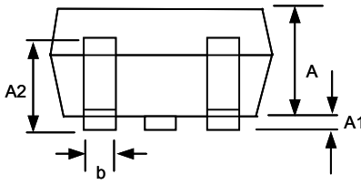
SOT 23 (T7) Package
