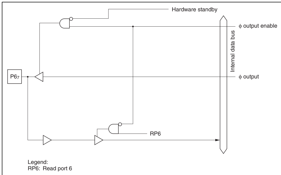
Figure C.2 (d) Port 6 Block Diagram (Pin P6 n )
