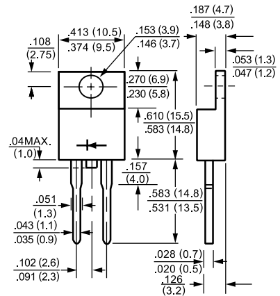
TO-220A
