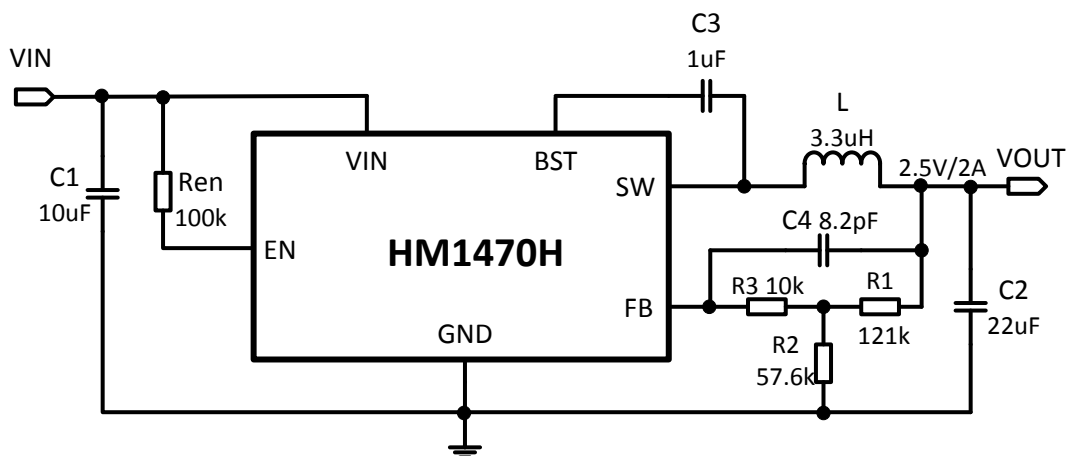
Figure5. 12V VIN, 2.5V/2A
