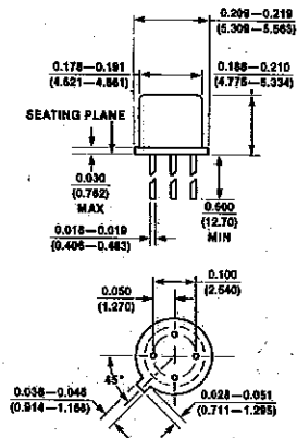
TO-72 (US)
