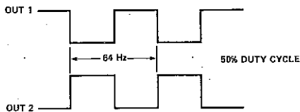
ICM 7051A
