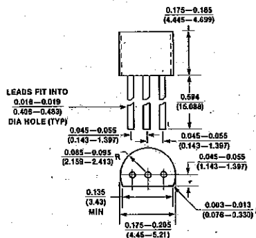
TO-92 (ZR)
