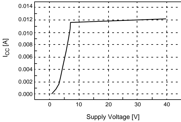
V_{CC}-I_{CC}
