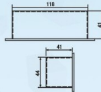
名称: 控制面板 型号: WD-02L CONTROL PANEL MODEL: WD-02L
