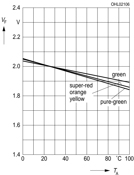
Durchlaßspannung V_F = f(T_A) Forward voltage I_F = 10 \text{ mA}
