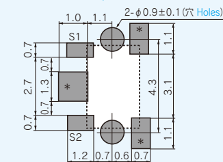
推奨はんだ付けパターン Recommendable soldering pattern
