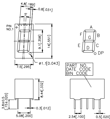
A. LTS-360/367
