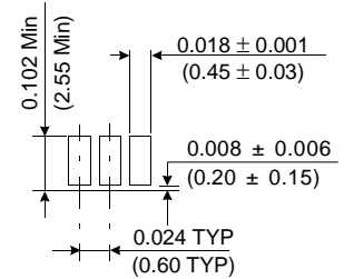
Detail Y
