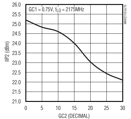
IIP2 vs. GC2
