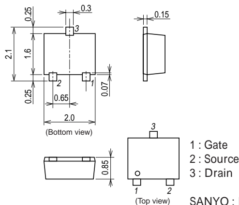
外形図 2167A
