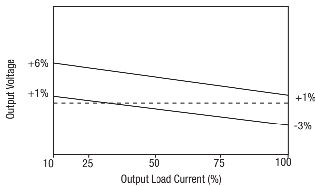
15V Output
