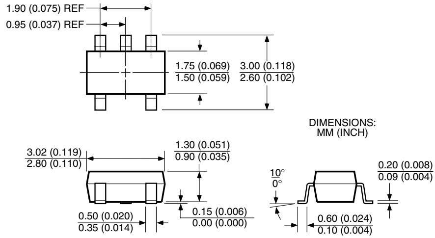
SOT-23-5 (M5)
